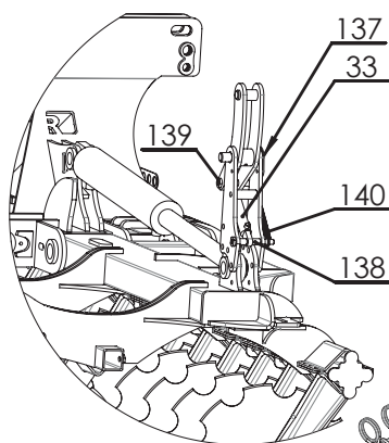
Hydrauliczna blokada ramion w pozycji transportowej Hydraulic arm lock for transport position
