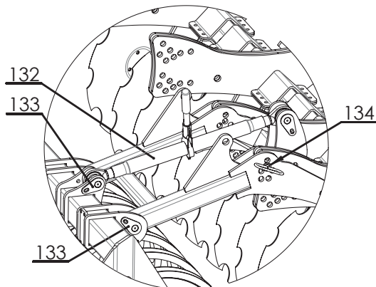
Wał tandem U-ring Ø540 Tandem U-ring roller Ø540
