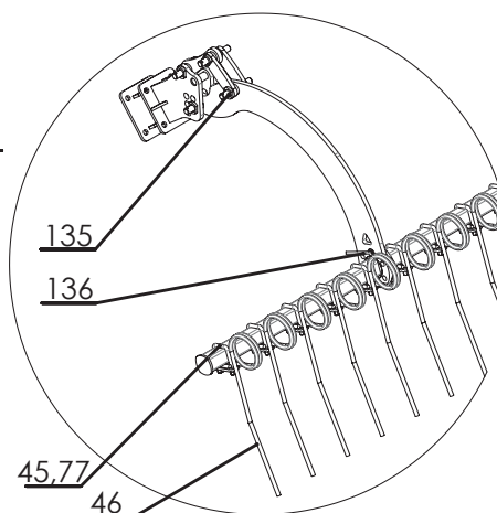
Wersja zawieszana Mounted version
