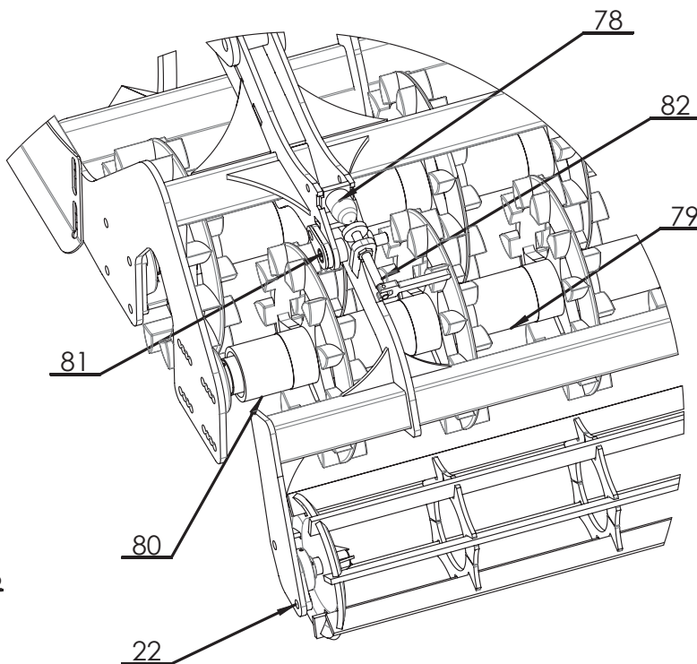
Wał Tandem Crosskill Ø400 + wał Finisher Tandem Crosskill roller Ø400 + Finisher roller
