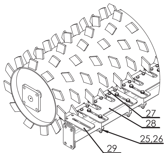
Wał Packer Ø460 Packer roller Ø460
