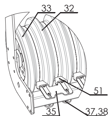
Wał gumowy Ø500 dla wersji 3,0m
