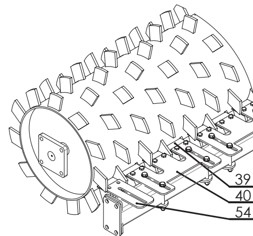
Wał Packer Ø460/550
