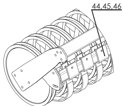
Wał U-ring Ø540 Wał T-ring Ø500 Ø600
