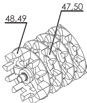
Wał CROSSKILL Ø400 Ø500
